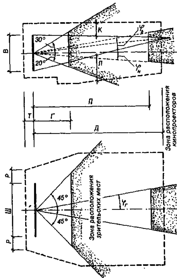
Параметры зрительского зала и киноэкрана при кинодемонстрации
