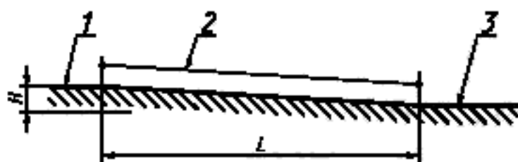
1 — горизонтальная площадка; 2 — наклонная поверхность пандуса; 3 — горизонтальная площадка
